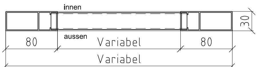
Schnitt A-A
