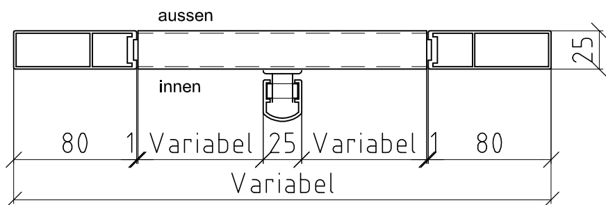
Schnitt A-A
