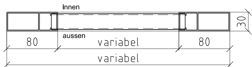
Schnitt A-A
