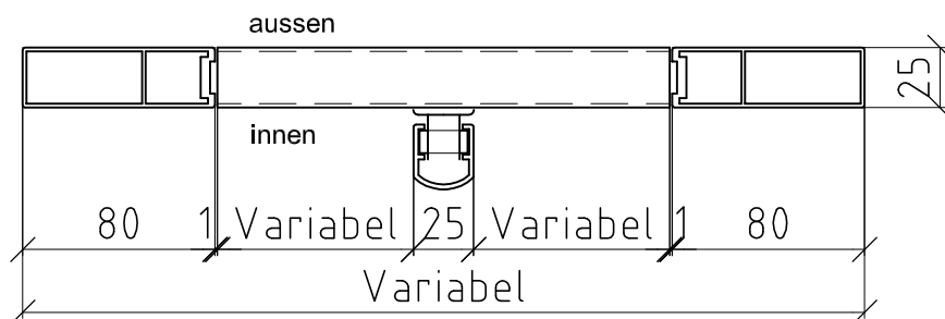
Schnitt A-A
