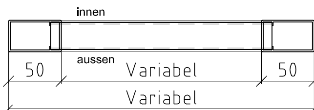
Schnitt A-A
