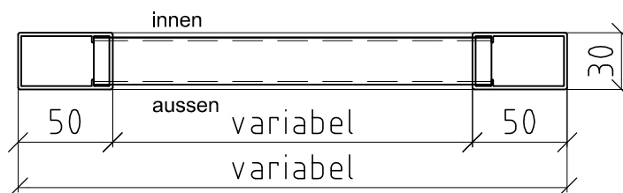
Schnitt A-A
