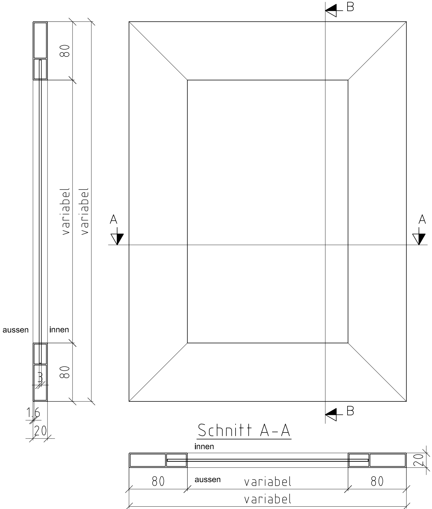
Schnitt B-B
